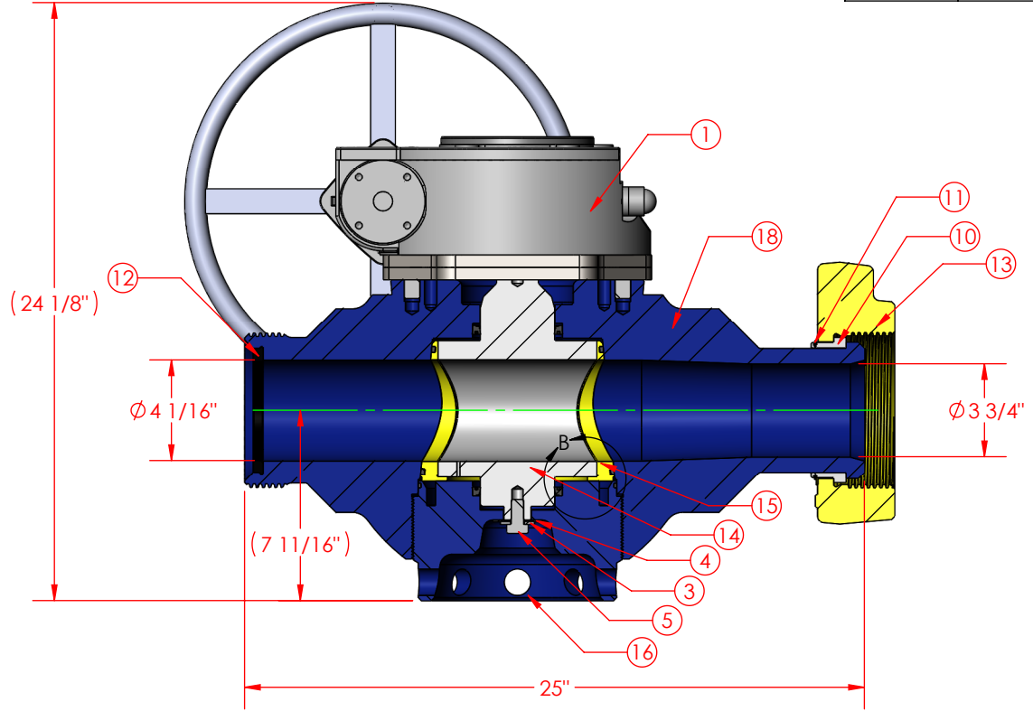
SECTION A-A
